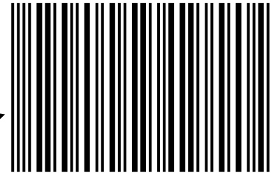
I 2of5
